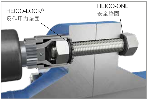
在通孔上使用HEICO-LOCK® 反作用力垫圈和HEICO-ONE安全垫圈
